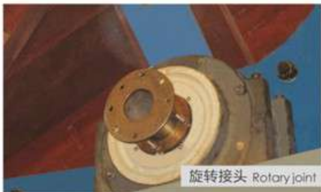
鼓体内结构 Inside drum
